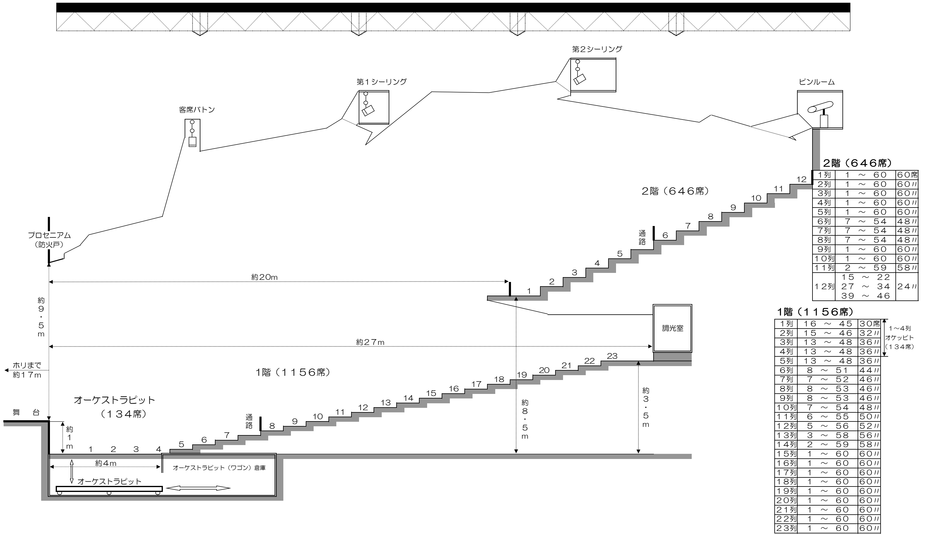
新宿文化センター 大ホール 客席断面図
