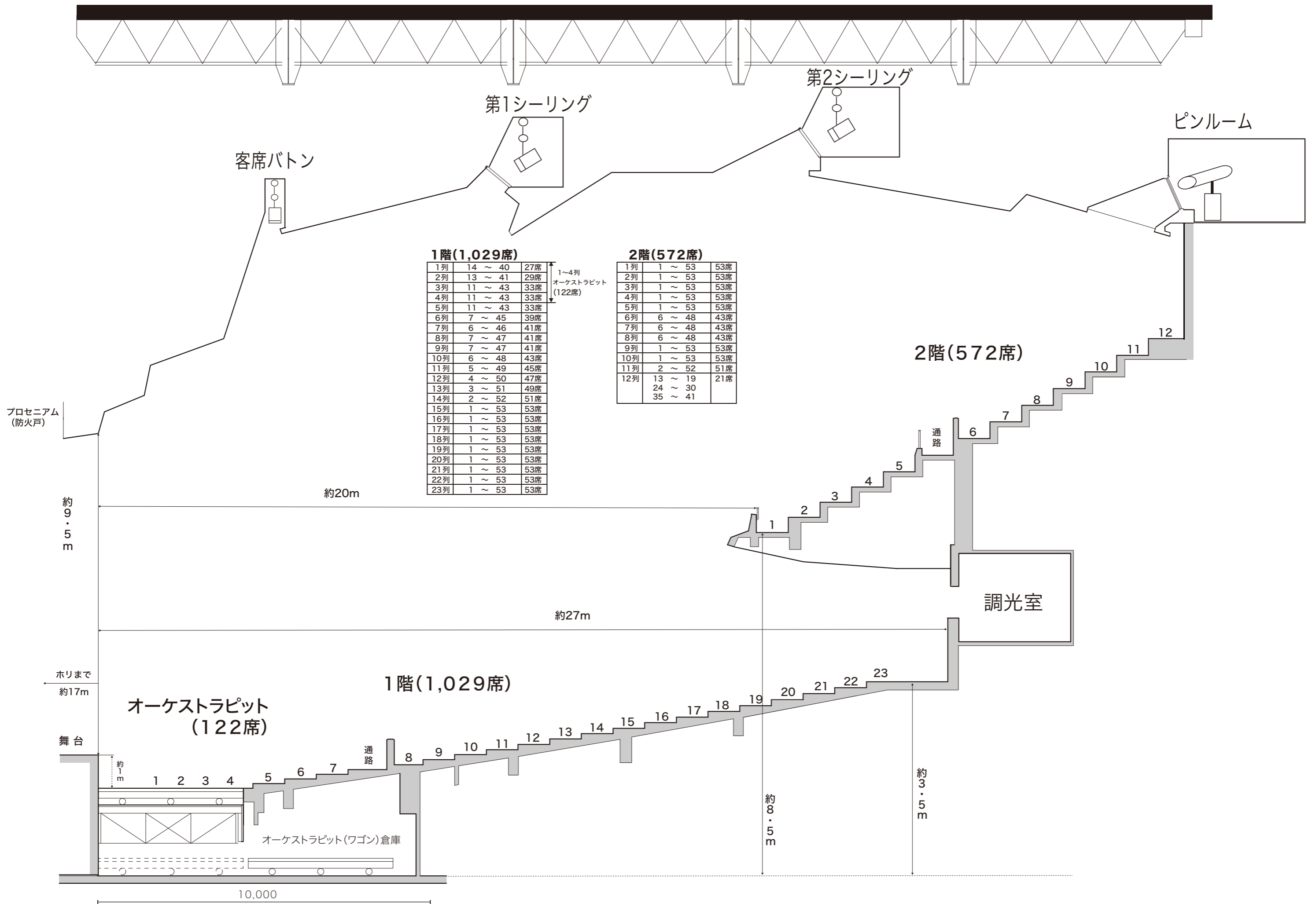
大ホール 客席断面図
